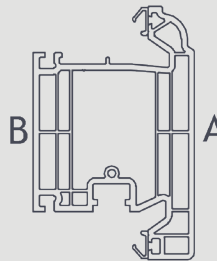
705541 Door Sash Open Out
